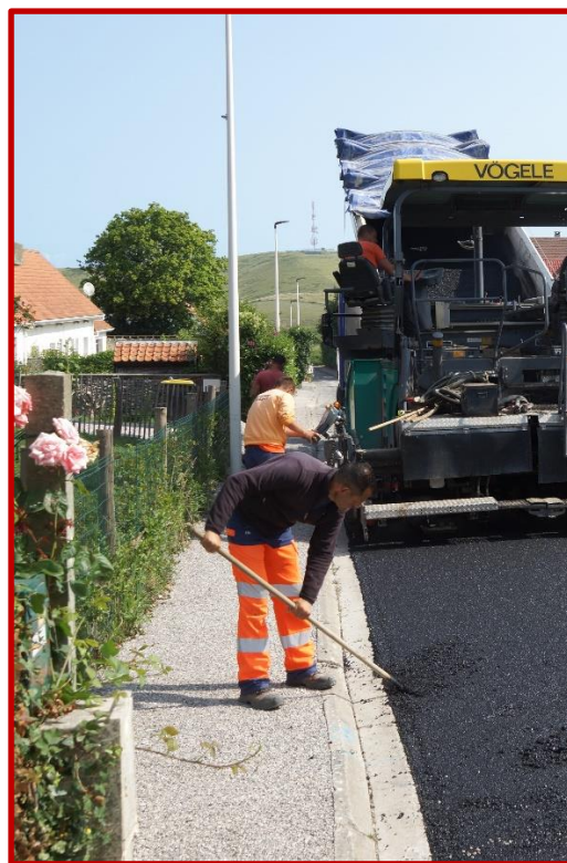
Nouvelles bordurations et réfection de la chaussée et des trottoirs
